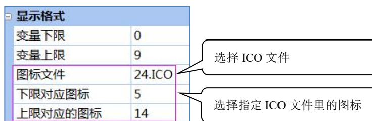
图 7-5-5 图标的引用
