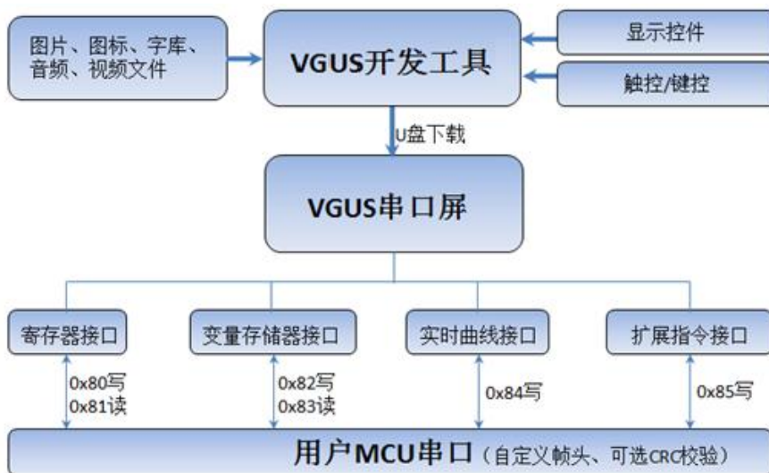
图 1-2-2 VGUS 屏系统架构
