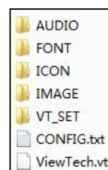
图 7-3-3 项目文件夹
